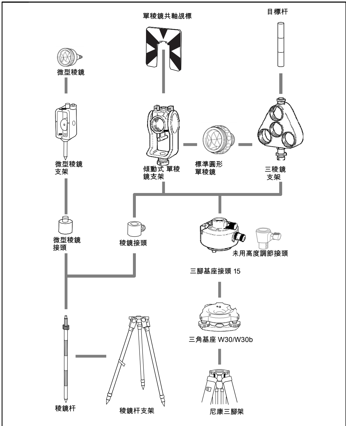
圖 8.2 稜鏡反射器側
