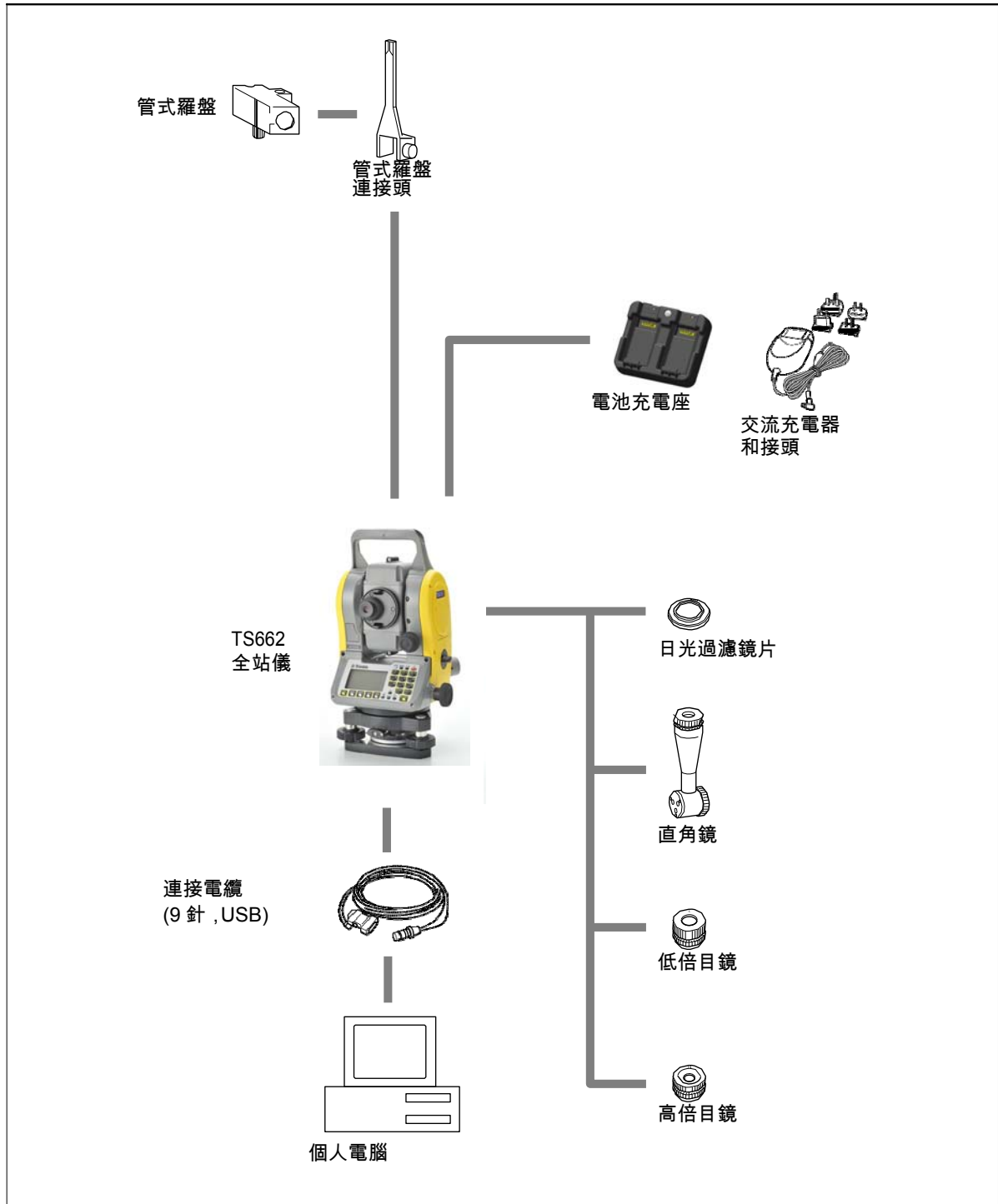
圖 8.1 測量主機側
